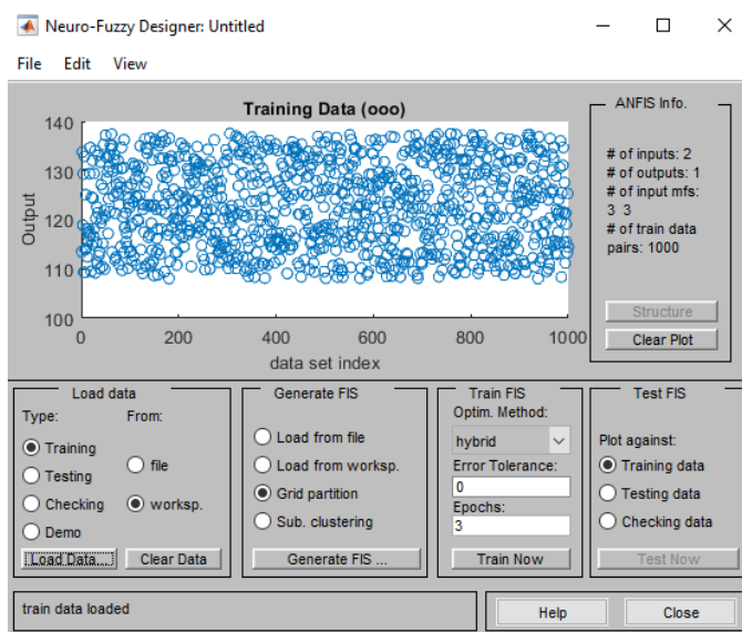
Рис.2. Обучение системы
